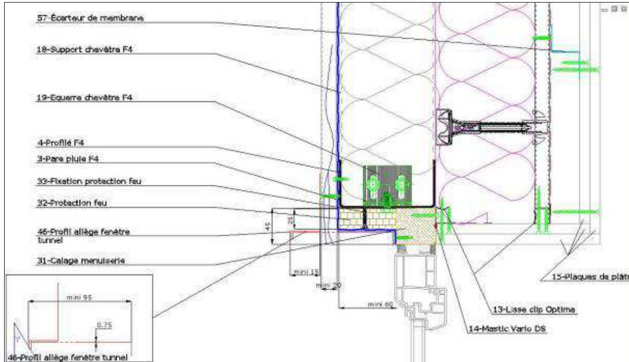
Traitement feu des baies pose en tunnel - Partie haute
