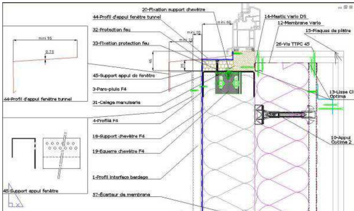
Traitement feu des baies pose en tunnel - Partie basse
