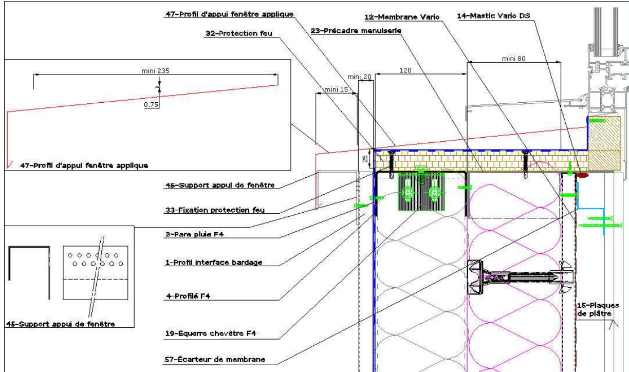
Traitement feu des baies en applique – Partie basse
