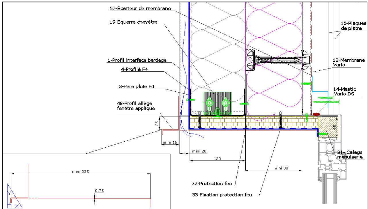
Traitement feu des baies pose en applique – Partie haute
