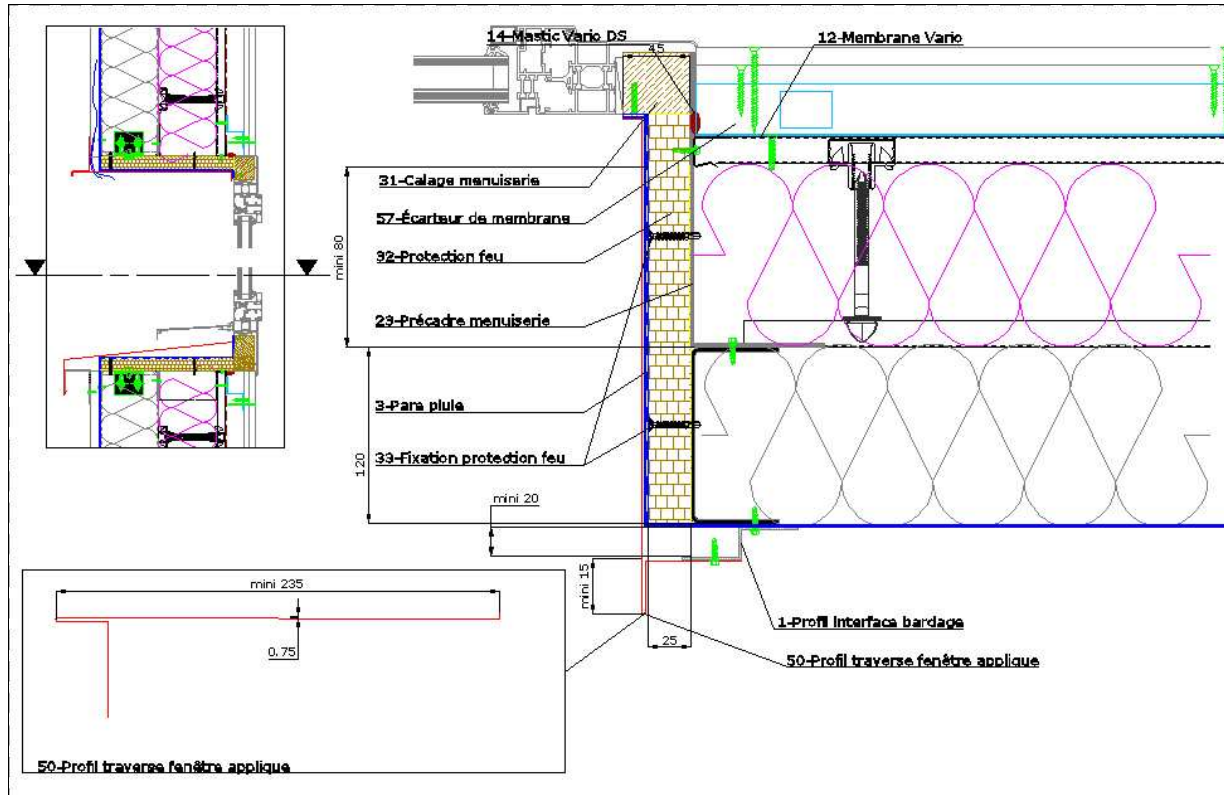
Traitement feu des baies pose en applique – Parties latérales
